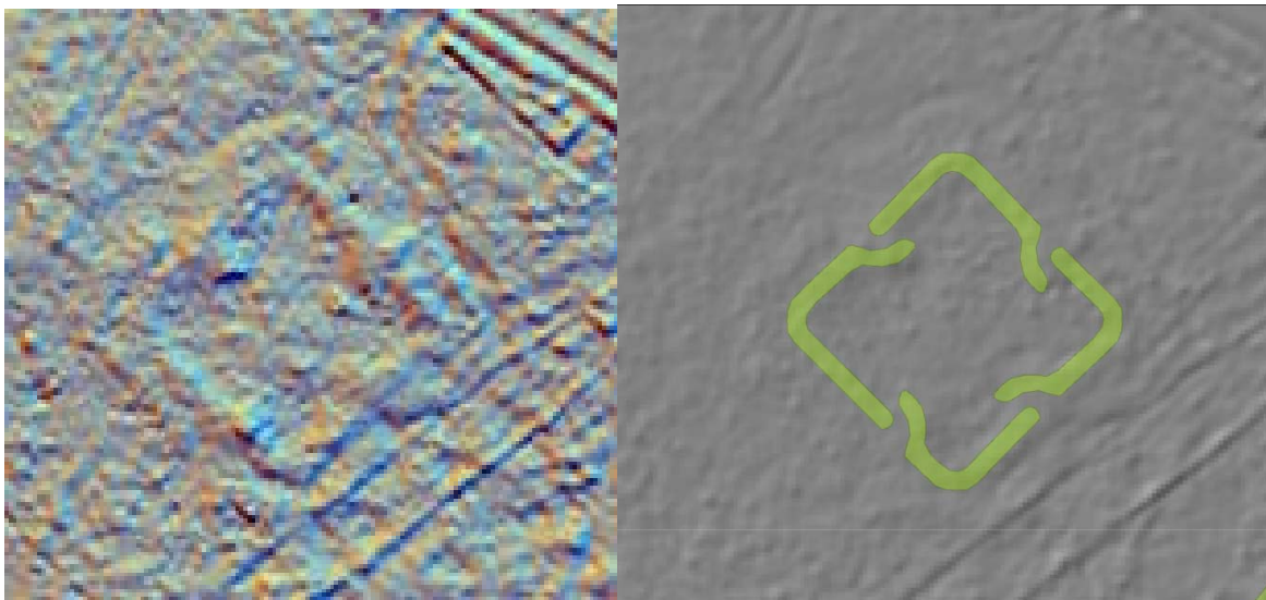
Abb. 2 Aifter. Römisches Übungslager Dürrenbruch 3 in unterschiedlichen Bearbeitungen im Laserscan (grün – Umzeichnung des inneren Walls).
