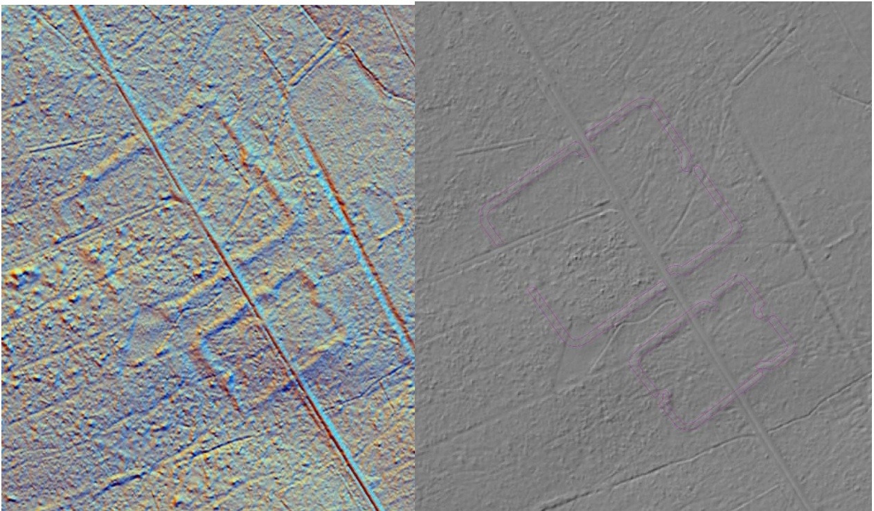
Abb. 2 Alfter. Römische Übungslager Pfaffenmaar 1 (nordwestliche) und 2 (südöstlich) in unterschiedlichen Bearbeitungen im Laserscan (pink – Umzeichnung des inneren Walles).
